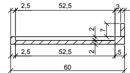
CORTE B-B
