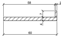
CORTE A-A
